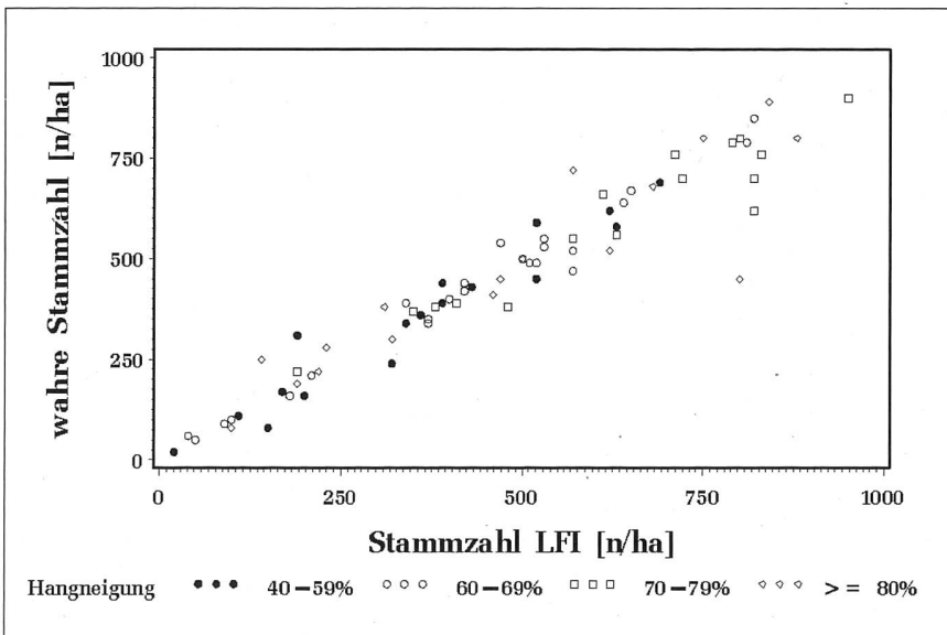
Abbildung 7: Stammzahl LFI versus wahre Stammzahl nach Neigungsklasse.
