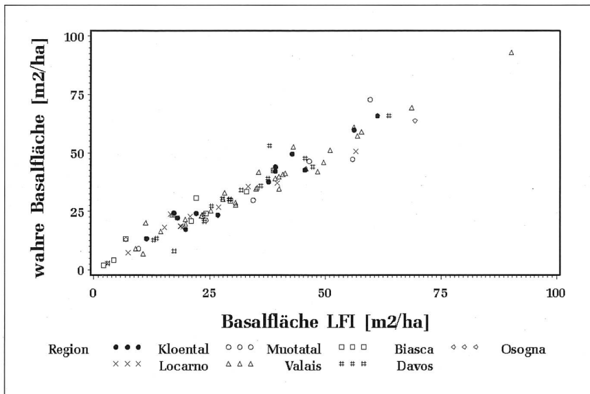
Abbildung 4: Basalfläche LFI versus wahre Basalfläche nach Region. Figure 4: NFI basal area versus true basal area according to region.
