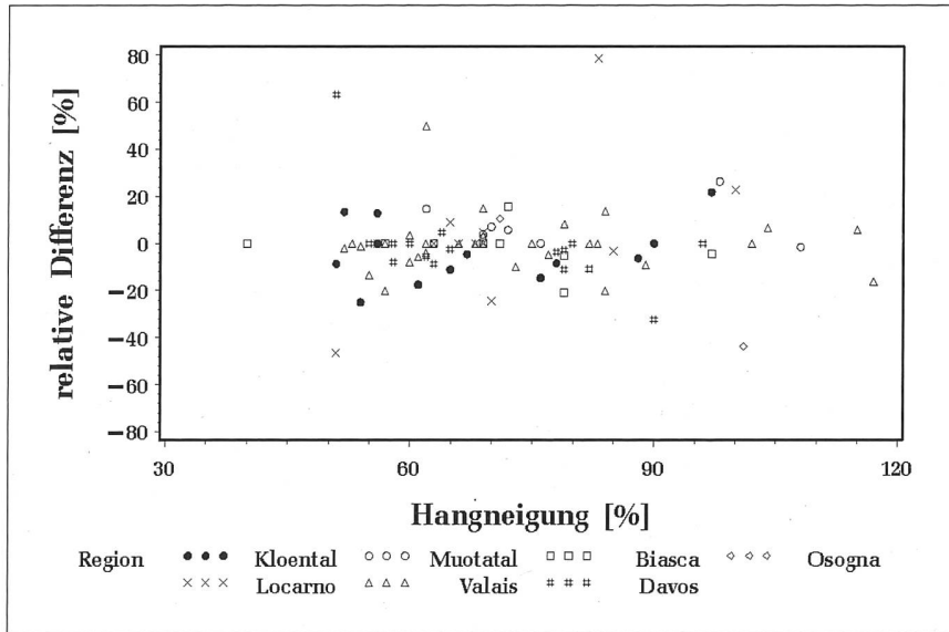
Abbildung 13: Relative Differenz der Stammzahlschätzung in Bezug auf die Hangneigung.
