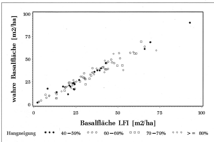
Abbildung 5: Basalfläche LFI versus wahre Basalfläche nach Neigungsklasse. Figure 5: NFI basal area versus true basal area according to slope class.
