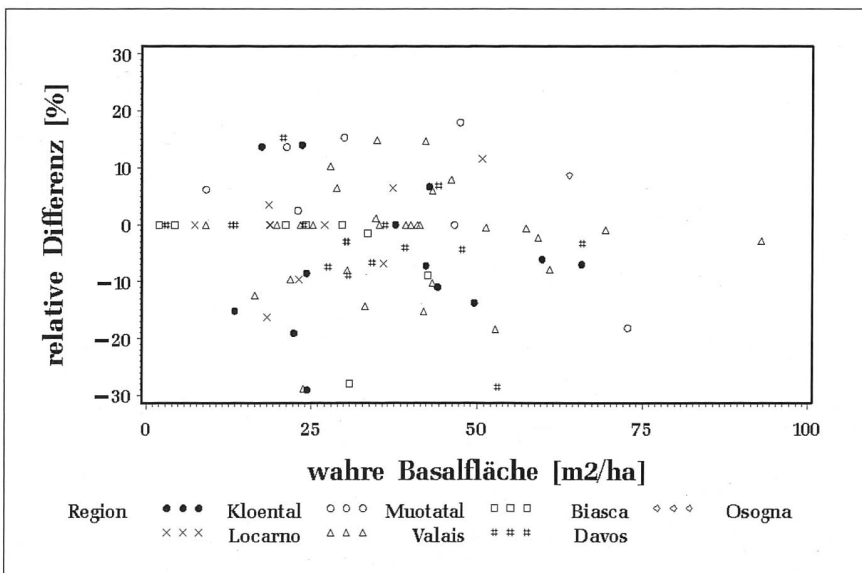
Abbildung 8: Relative Differenz der Basalfläche versus wahre Basalfläche nach Region.
