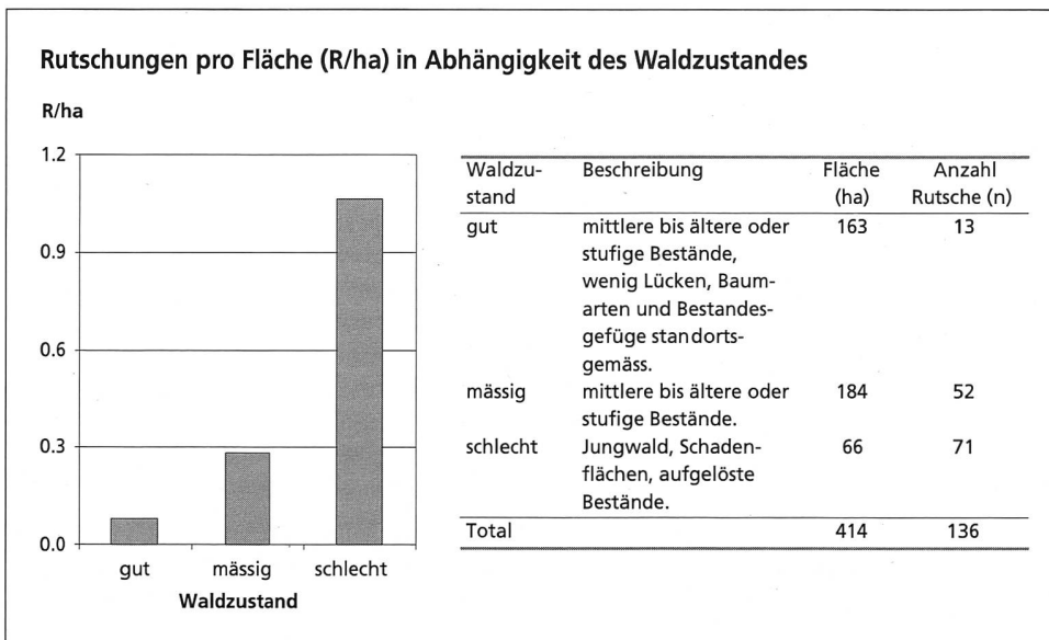
Abbildung 10: Waldzustand und Rutschungen (nach RICKLI et al. , 2000, Abbildung 6 ).
