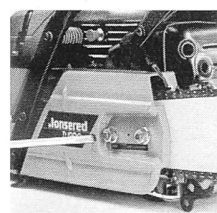
Seitliche Ketten- schnellspannung
