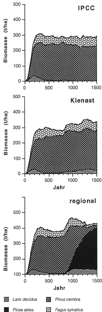
Abbildung 5: Simulierte Walddynamik unter den drei Klimaszenarien (Tabelle 2) am Standort Bever unter der Annahme, dass nur der heute vorhandene Artensatz zugelassen wird und die Verjüngung keinen klimatischen Einschränkungen unterworfen ist («Eliminationsszenario»). Jahre 0 bis 800: heutiges Klima; Jahre 800 bis 900: lineare Klimaveränderung. Jahre 900 bis 1500: konstantes, zukünftiges Klima (Tabelle 2).
