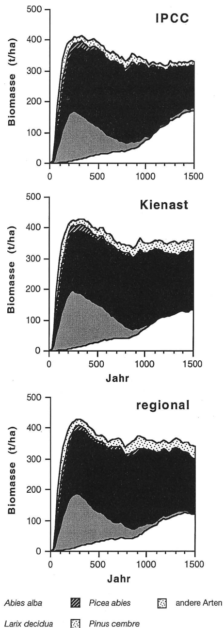
Abbildung 6: Simulierte Walddynamik unter den drei Klimaszenarien (Tabelle 2) am Standort Davos unter der Annahme, dass nur der heute vorhandene Artensatz zugelassen wird und die Verjüngung keinen klimatischen Einschränkungen unterworfen ist («Eliminationsszenario»). Jahre 0 bis 800: heutiges Klima; Jahre 800 bis 900: lineare Klimaveränderung. Jahre 900 bis 1500: konstantes, zukünftiges Klima (Tabelle 2).
