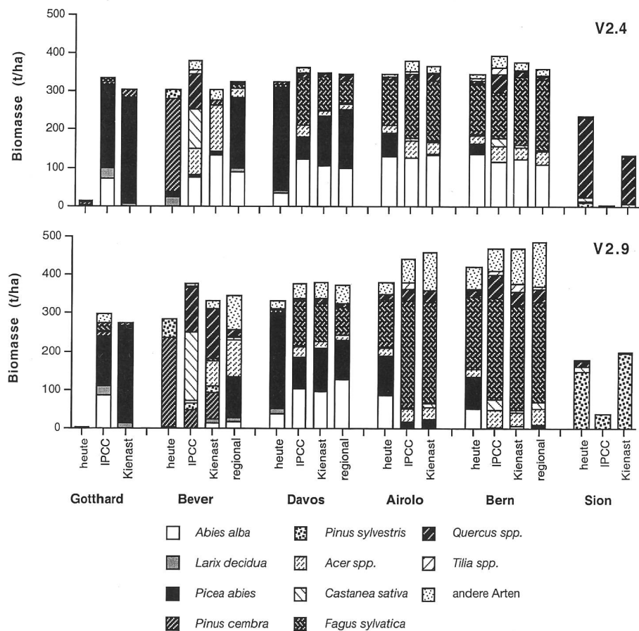
Abbildung 2: Simulierte Artenzusammensetzungen und oberirdische Biomassen im Gleichgewicht mit dem heutigem Klima («heute») und den drei Klimaszenarien für das Jahr 2100 (Tabelle 2) an sechs Standorten entlang einem Klimagradienten in der Schweiz (vgl. Tabelle 1). Oben: Modellversion FORCLIM 2.4 (BUGMANN, 1994, 1996, 1997; FISCHLIN et al. , 1995); unten: Modellversion FORCLIM V2.9 (BUGMANN & SOLOMON, 1999).
