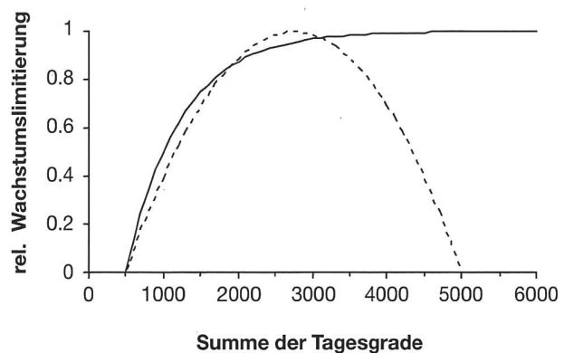
Abbildung 1: Beispielhafter Vergleich der relativen Wachstumslimitierung durch die Temperatur (hier wiedergegeben als Summe der Tagesgrade) in FORCLIM V2.9 (ausgezogene Kurve) mit der parabolischen Funktion, die in vielen anderen Modellen (u.a. FORCLIM V2.4) verwendet wird (gestrichelte Linie). Die Schnittpunkte der parabolischen Funktion mit der x-Achse werden üblicherweise mit den nördlichen bzw. südlichen Verbreitungsgrenzen gleichgesetzt (vgl. SHUGART, 1984), so dass dieses Modell an der südlichen Verbreitungsgrenze Nullwachstum produziert, während die in FORCLIM V2.9 verwendete Funktion dort die geringste temperaturbedingte Wachstumslimitierung simuliert (vgl. BUGMANN & SOLOMON, 1999).
