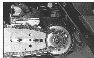
Innenliegende Kupplung Softstart
