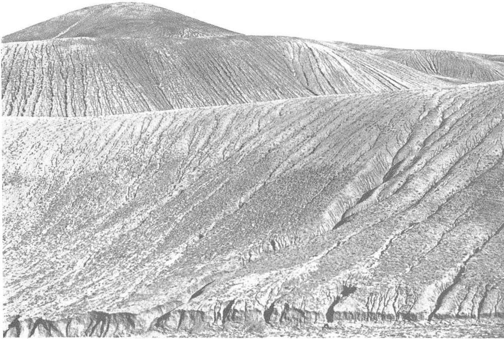
Bild 2. S.-Kalifornien. Grabenerosion.
