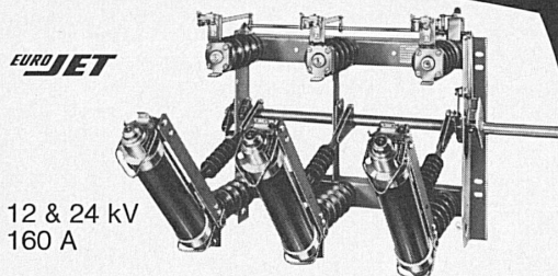
Sicherungs-Lasttrennschalter mit autoneumatischer Blasung, 3-polig, Typ BB, für vertikale Innenmontage gemäss Normen SEV - CEI - VDE
