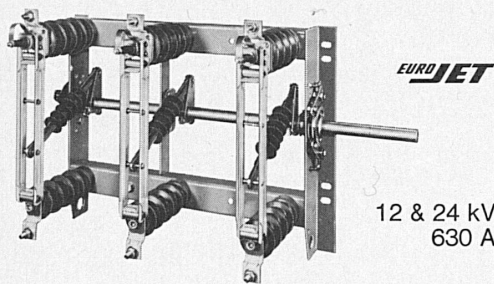
Lasttrennschalter mit autoneumatischer Blasung, 3-polig, Typ CC für vertikale Innenmontage gemäss Normen SEV - CEI - VDE
