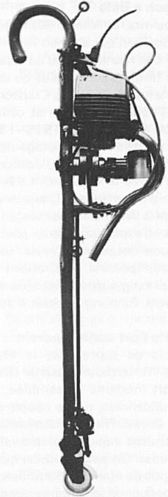
Spazierstock, motorisiert
