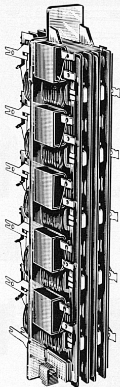
Baueinheit: Relaisstreifen mit 5 ESK-Relais natürliche Grösse
