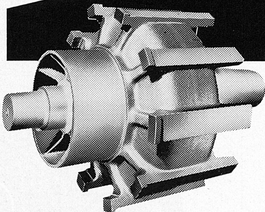
Rotor, in zwei Teilen gegossen und zusammenschweisst, Gewicht 380 kg
