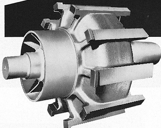
Rotor, in zwei Teilen gegossen und zusammengeschweisst, Gewicht 380 kg
