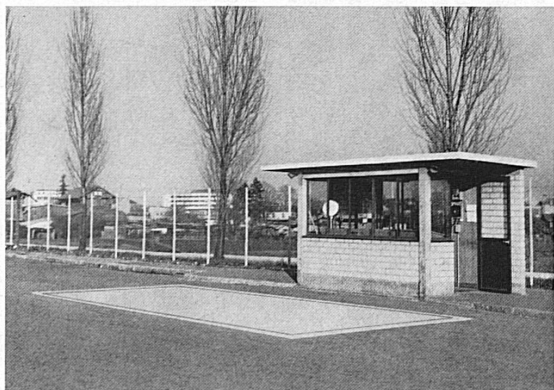
Abbildung: Fahrwerkswaage 40 000 kg Brückengröße 10 x 3,2 m Laufgewichtsbalken mit Messkopf kombiniert
