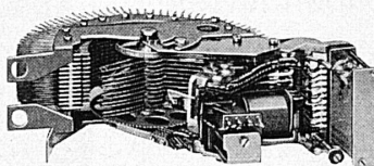
Motorwähler neuester Bauart
