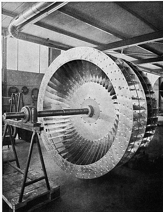
Doppel-Ventilatorrad in Aluminium für 120 000 m 3 /h
