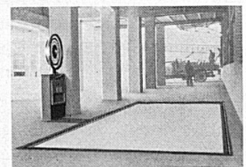
Brückenwaage für Straßenfahrzeuge. Wägefähigkeit 30 000 kg mit automatischer Gewichtsanzeige und Registrierung
