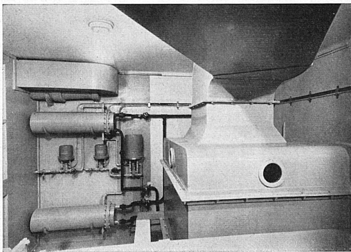
Klima-Anlage
