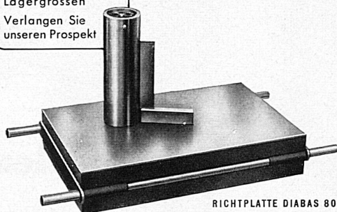
RICHTPLATTE DIABAS 800 Kontrolle eines Winkels mit Messzylinder
