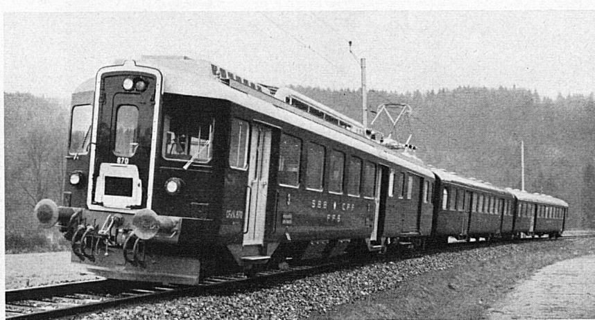
SBB-Pendelzug bestehend aus Triebwagen CFe 4/4, Zwischenwagen C4ü und Steuerwagen BCt4ü
