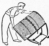
Faßbock mit Abwälzkufen für Einmannbetrieb
