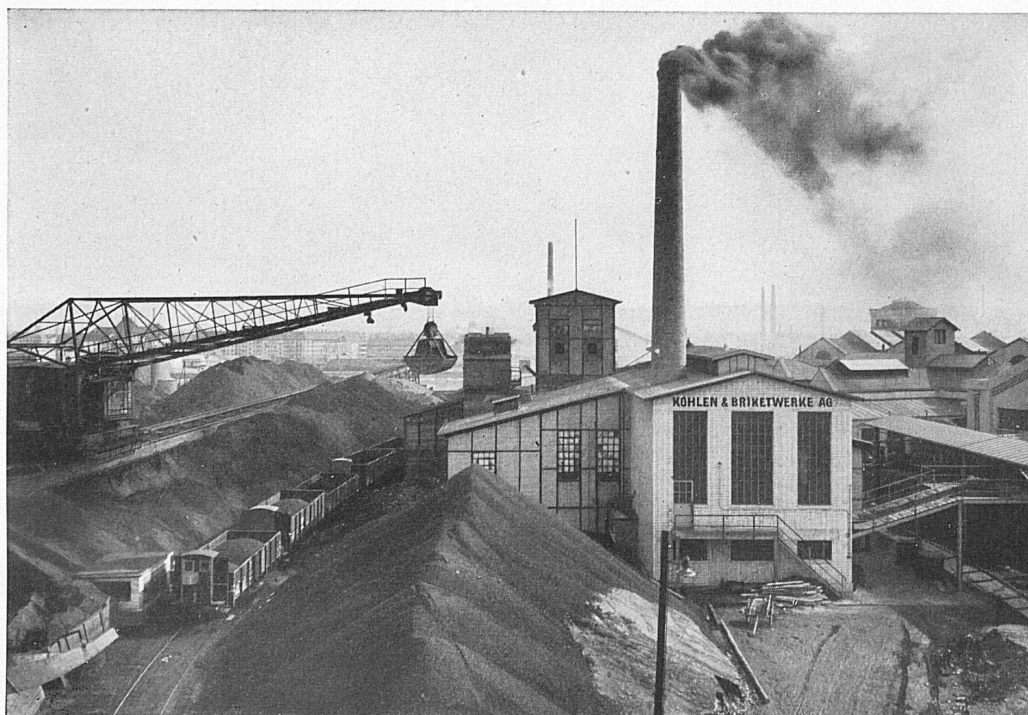
Vorderansicht der Brikettfabrik im Rheinhafen St. Johann
