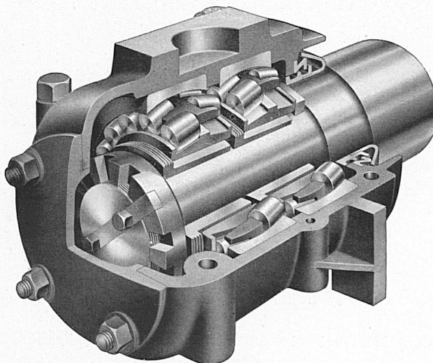
Achsbochse mit Pendelrollenlagern
