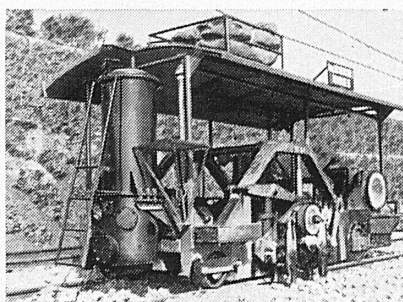
Bourreuse
