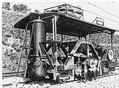
Bourreuse
