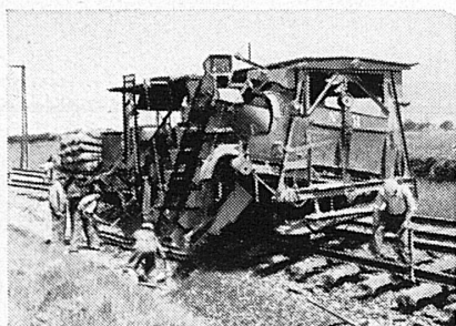
Cribleuse
