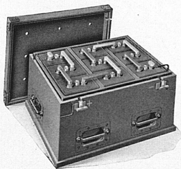
Batterie Type SBB 18 Volt, 100 Ah
