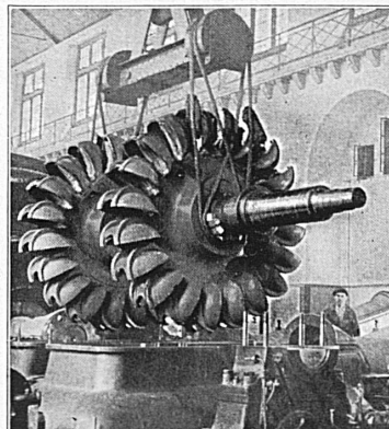
Rotor einer 15000-PS-Turbine Kraftwerk Amsteg der SBB
