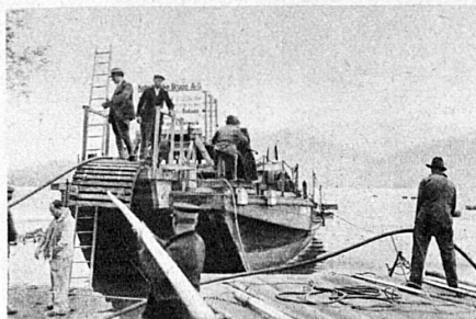
Verlegung eines Telefonkabels von 2620 m (in einer Länge) und 30 Tonnen Bruttogewicht durch den oberen Zürichsee zwischen Rapperswil und Lidwil (Schwyz) - Einzelwerk - für die Schweiz. Bundesbahnen. 17. Aug. 1937. Anknüpft des Verlegeschiffes in Rapperswil
