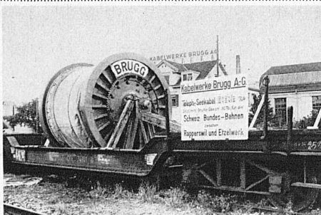
Verlegung eines Telephonkabels von 2620 m (in einer Länge) und 30 Tonnen Bruttogewicht durch den oberen Zürichsee zwischen Rapperswil und Lütwil (Schwyz) — Einzelwerk — für die Schweiz, Bundesbahnen. 17. Aug. 1937. Das spezialisierte, auf eiserner Spezialtrammel aufgewickelte Kabel auf dem Fabrikgeleise der Kabelwerke Brugg AG.
