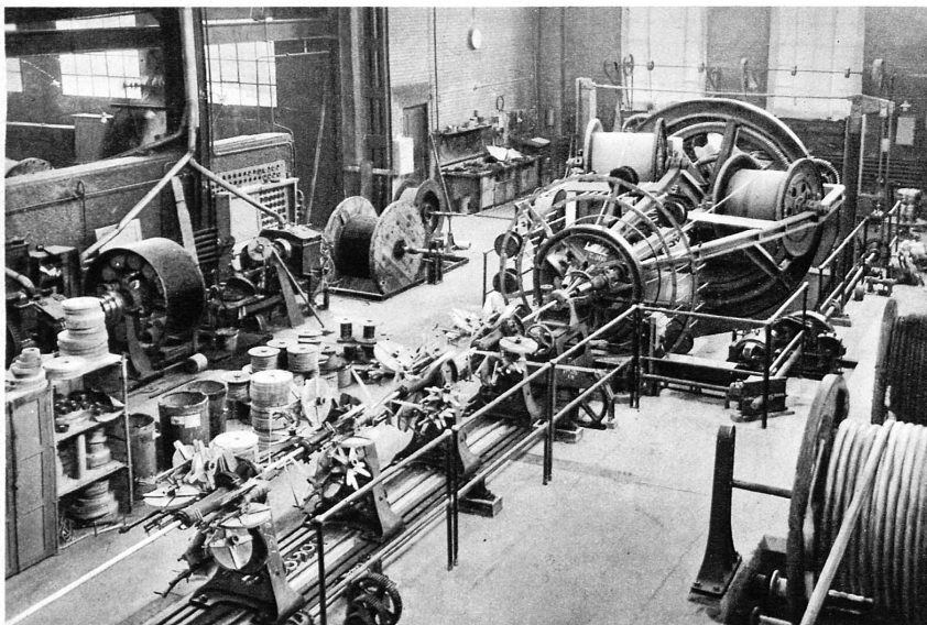
Blick in eine Fabrikations-Abteilung mit Hochspannungs-Verseilmaschine
