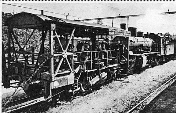
Zahnstangen geliefert von der Giesserei Bern der Ludw. von Roll'schen Eisenwerke
