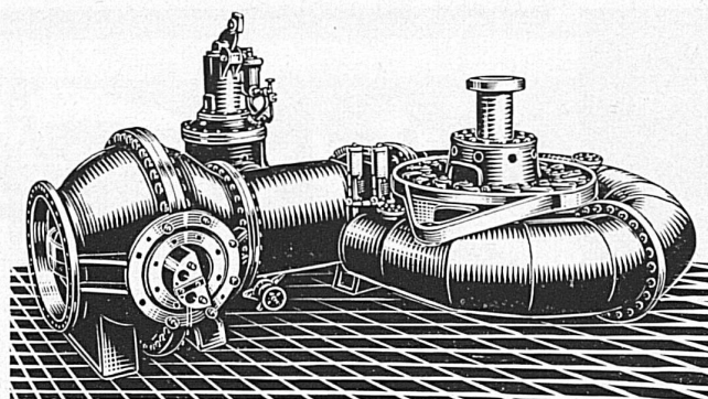
Francis-Spiral-Turbine von 10240 PS-Leistung, mit Bell-Patent-Kugelschieber, nebst einer weiteren Turbine von 4000 PS, für das neue, vollautomatische Kraftwerk Kaiserstuhl der C.K.W., Luzern
