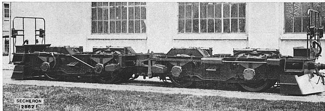
5 Locomotives à courant continu type B 0 -B 0 , 2x1200 et 2400 V, 920 ch pour le Chemin de Fer de St-Georges de Commiers à La Mure et à Gap (Isère) Truck à 4 moteurs jumelés et à transmission élastique, système Sécheron
