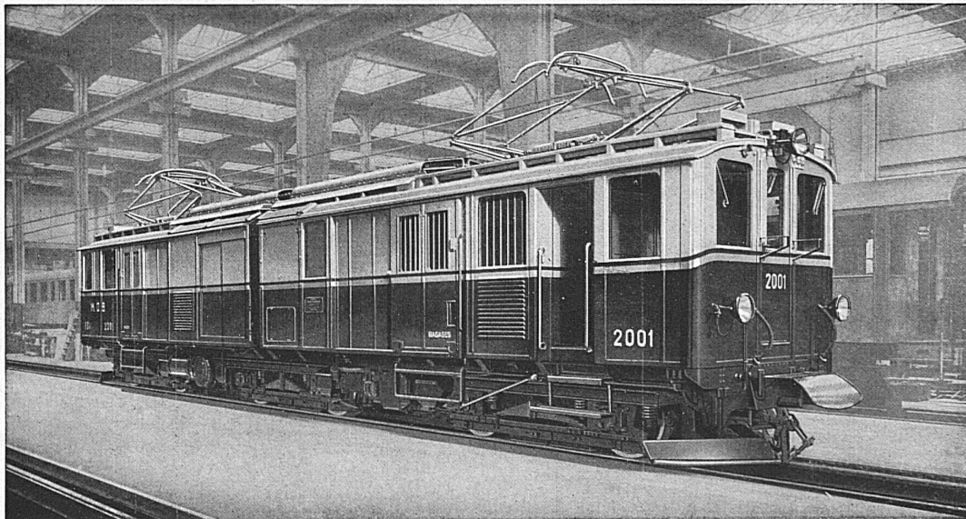
1000 HP Lokomotive der Montreux-Berner Oberland-Bahn
