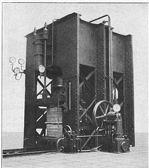
Hydraulische Plattenpresse für 4500 t Be- triebsdruck m. Presspumpe
