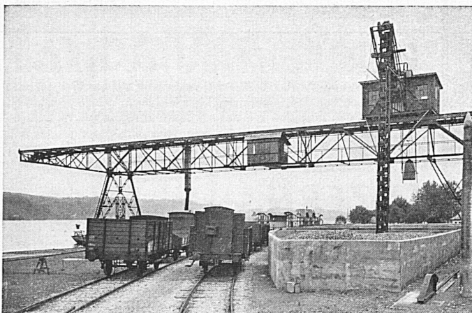
Kranbrücke einer Kies- und Sand-Verladeanlage
