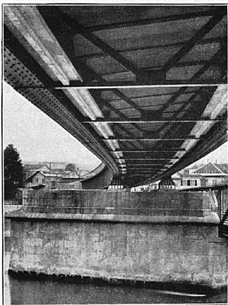
Neue Eisenbahnbrücke sog. „Gäubahnbrücke“ der SBB über die Aare bei Olten Erstellt 1927
