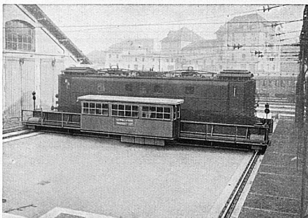
Elektrische Schiebebühne von 150 Tonnen Tragkraft, 18 Meter Grubenbreite, der Schweiz. Bundesbahnen, Kreis II, Luzern
