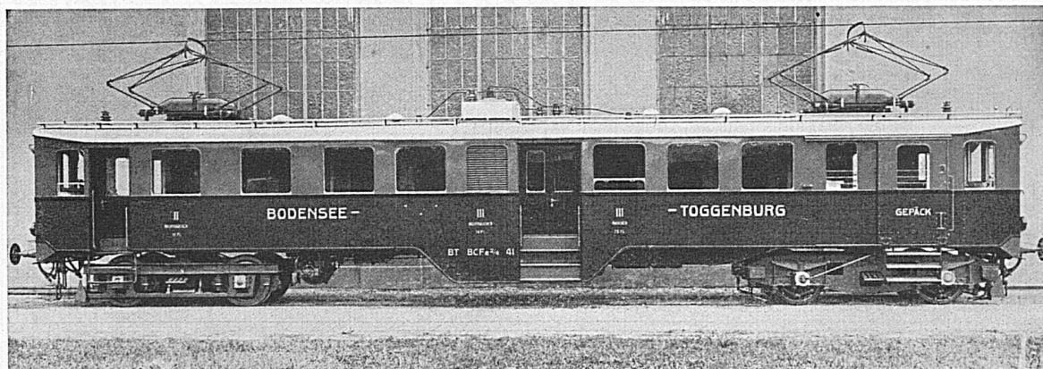
Chemin de fer du Lac de Constance au Toggenbourg (Bodensee-Toggenburg-Bahn) Automotrice type BCFe \frac{2}{4} de 900 ch à commande individuelle des essieux Système Sécheron
