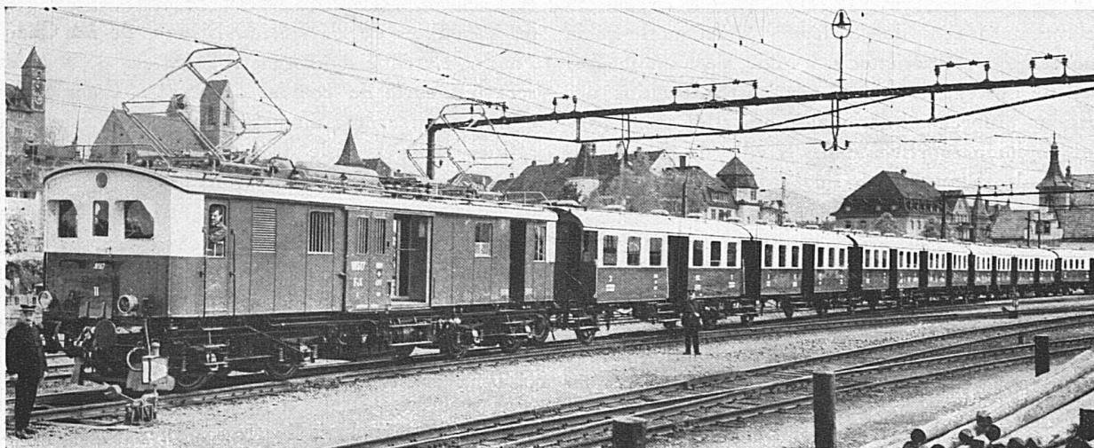
Train-navette „bleu et blanc“ à formation fixe, tiré par une automotrice Sécheron de 1100 ch; rive droite du lac de Zurich
