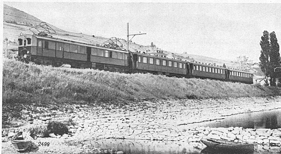
Train léger tiré par une automotrice de 1440 ch, vitesse maximum 90 km/h, ligne de Berne à Neuchâtel, environs de Saint-Blaise
