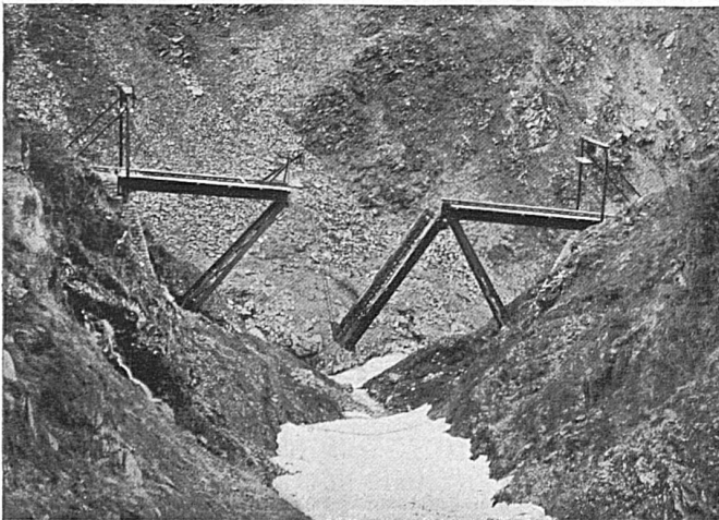
Steffenbachbrücke der Furka-Oberalp-Bahn - Diese Brücke wird jeden Winter wegen Lawinengefahr zusammengeklappt, auf die Widerlager zurückgelegt, und im Frühling wieder hochgezogen und zusammenmontiert
