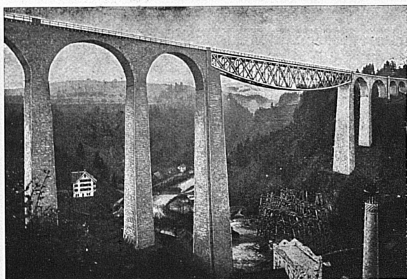
Sitterviadukt der Bodensee-Toggenburg-Bahn
