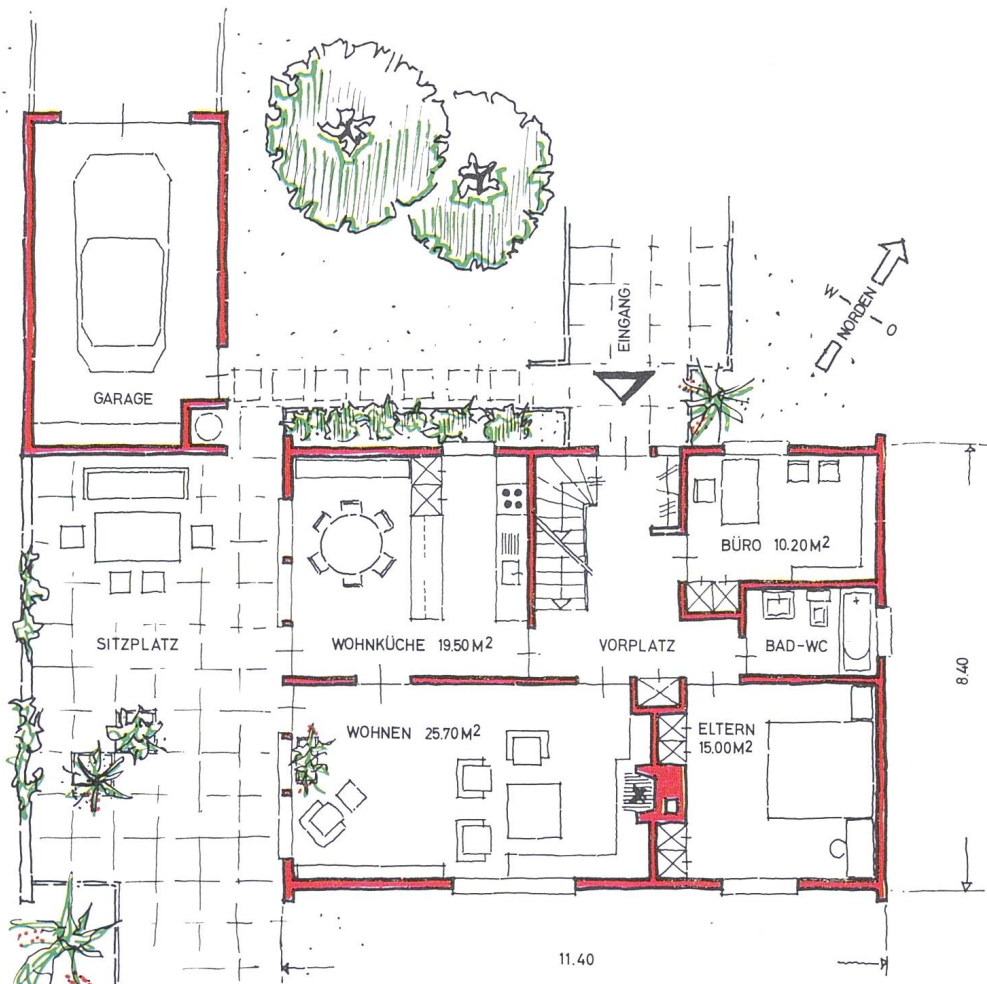
Hauptgeschoss Voll unterkellert
