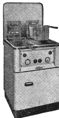
↑ Modell De-Rapide Masse: 60×60×88 cm, 2 Ölbassins zu je 12 l Inhalt Anschlusswert der 2 getrennten Heizungen je 6,2 kW Fr. 2650.—
