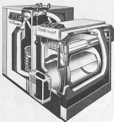
Hoval UnoLyT Niedertemperatur-Oel-/Gaskessel mit Beistellboiler Hoval CombiVal
