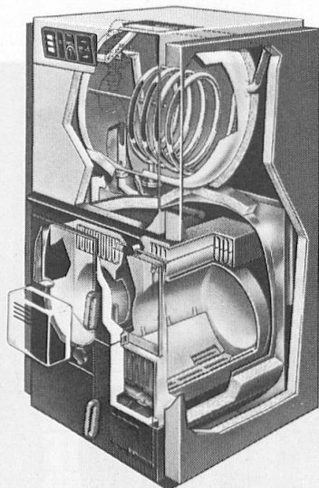
Hoval DuoLyT Niedertemperatur-Doppelkessel mit aufgebautem, vom Kessel getrennten Boiler
