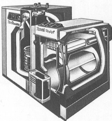
Hoval UnoLyt Niedertemperatur- Öel-/Gaskessel mit Beistellboiler Hoval CombiVal
