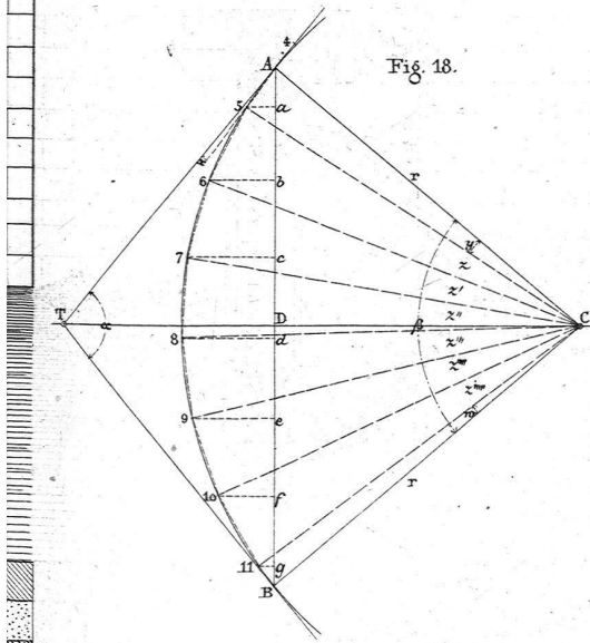
Methode zum Curven-Abstecken. Von Ganter
