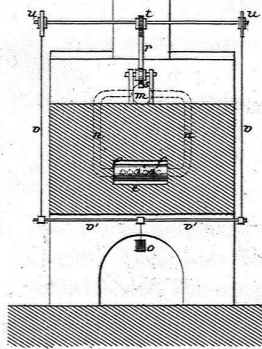
Fig. 3. Schnitt nach w-x
