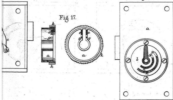
Sicherheits-Schlösser. Von Henderson
