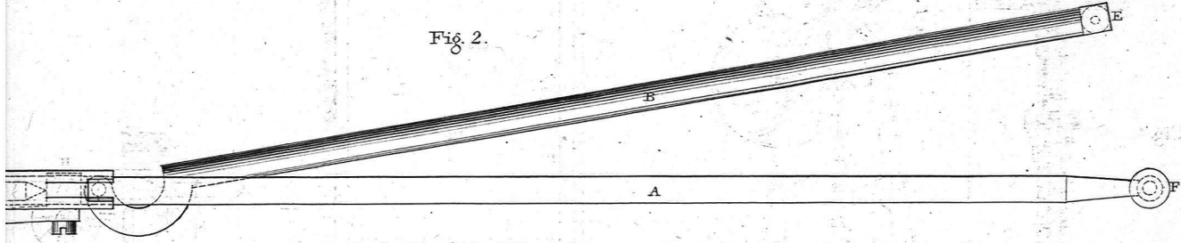
Libellen-Dezimalwaage von Pfanzeder. Maßstab 3/4.
