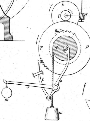
Mühle mit zwei bewegl. Steinen.
