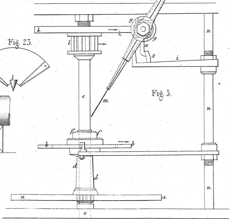
Weule's Thurmuhr mit Remontoir.
