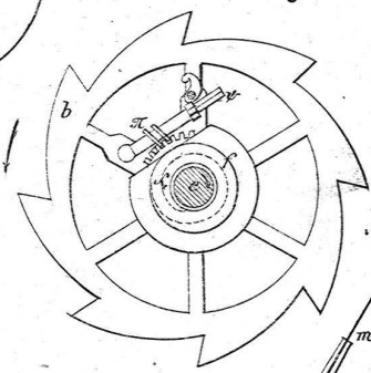
Weule's Thurmuhr mit Remontoir.
