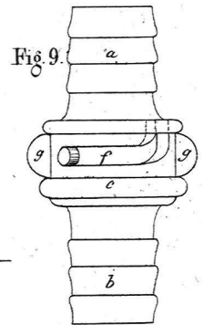
Schroter's Kuppelung für Spritzenschläuche.
