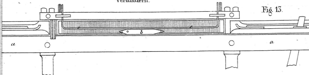
Ahler's Vorrichtung, das Herausfliegen der Weberschützen zu verhindern.
