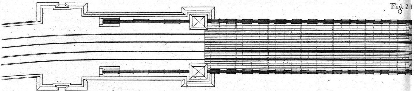
Erste versteifte Eisenbahn-Kettenbrücke über den Wiener Donaukanal. Nach Schnirch's System
