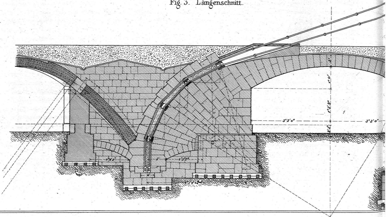
Erste versteifte Eisenbahn-Kettenbrücke über den Wiener Donaukanal. Nach Schnirch's System
