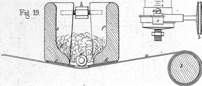
Werkzeug zum Noppen des Tuches.
