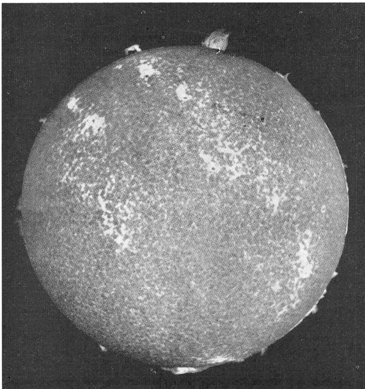
Sonne mit Protuberanzen (brennende Gaswolken)
