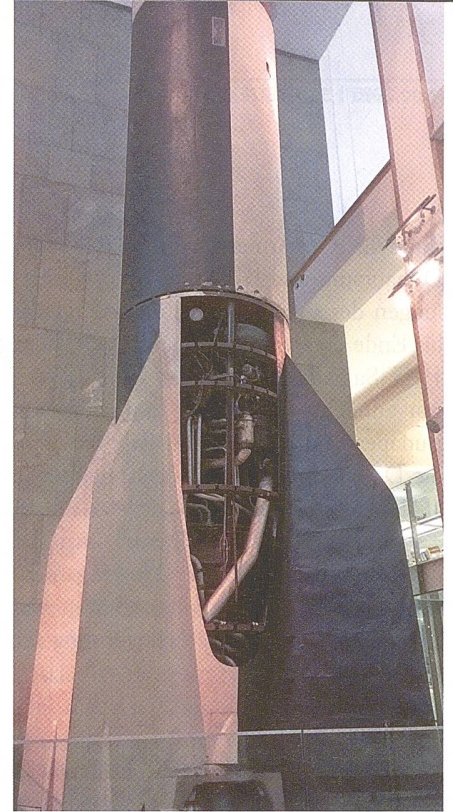
Das Waffensystem V 2 für den Fernbeschuss mit Raketen im Londoner Science Museum. Das Antriebsaggregat ist gut zu erkennen.
