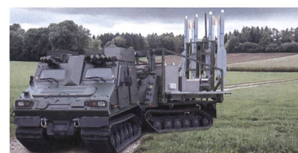
IRIS-T SLS auf Hägglunds BV-410.
